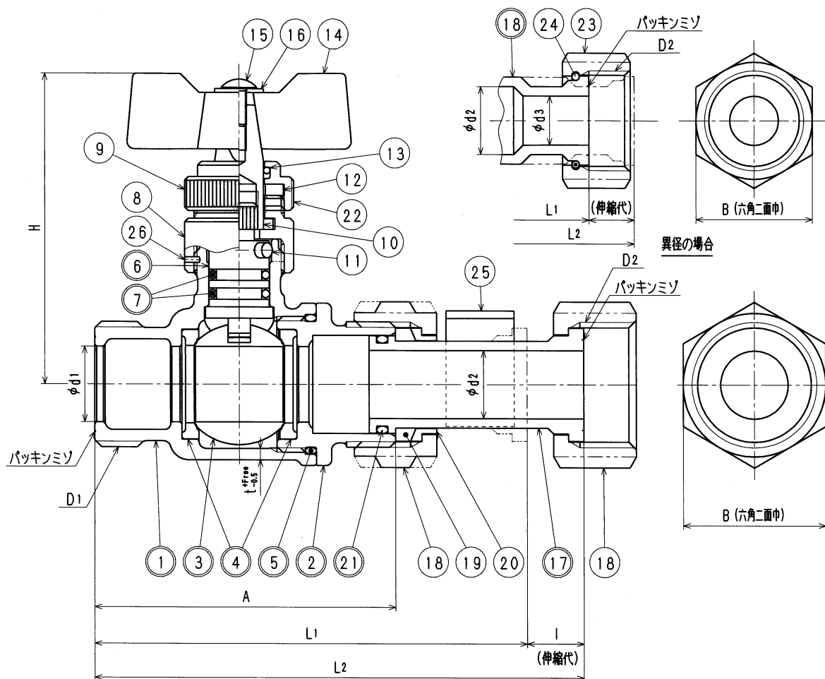
寸法表
